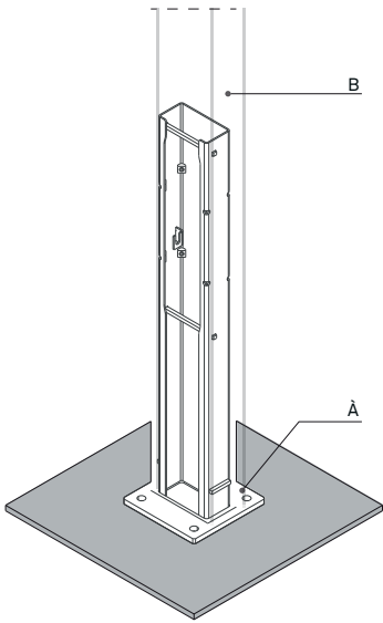
Fixation avec bride apparente
