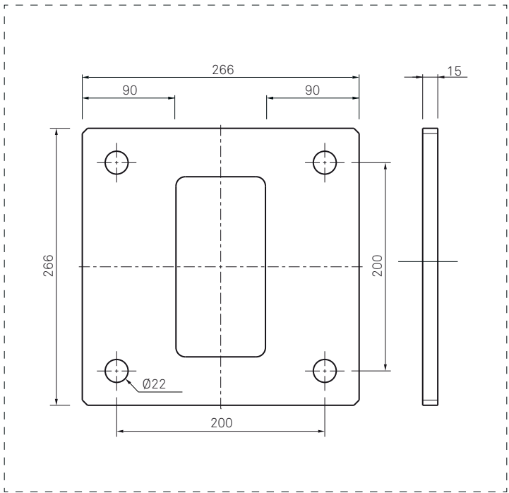
Détail de la bride - mesures en mm
