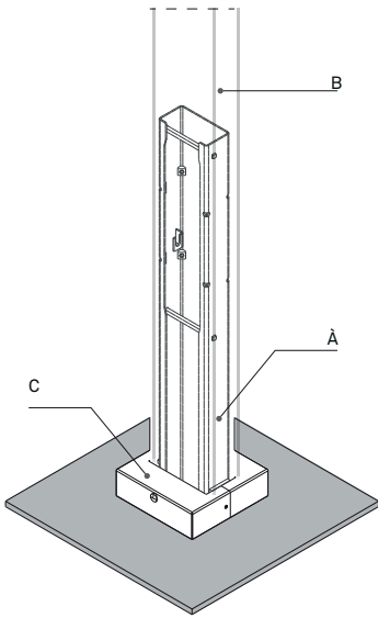
Fixation avec couvercle à bride
